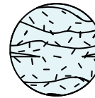
URANUS
