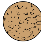
JUPITER
